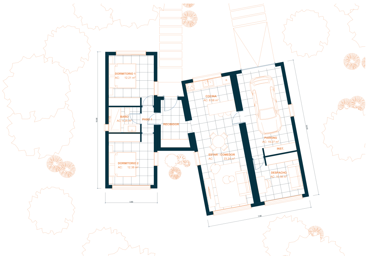
CASA RAÍCES · PLANTA BAJA · ESC. 1:50
