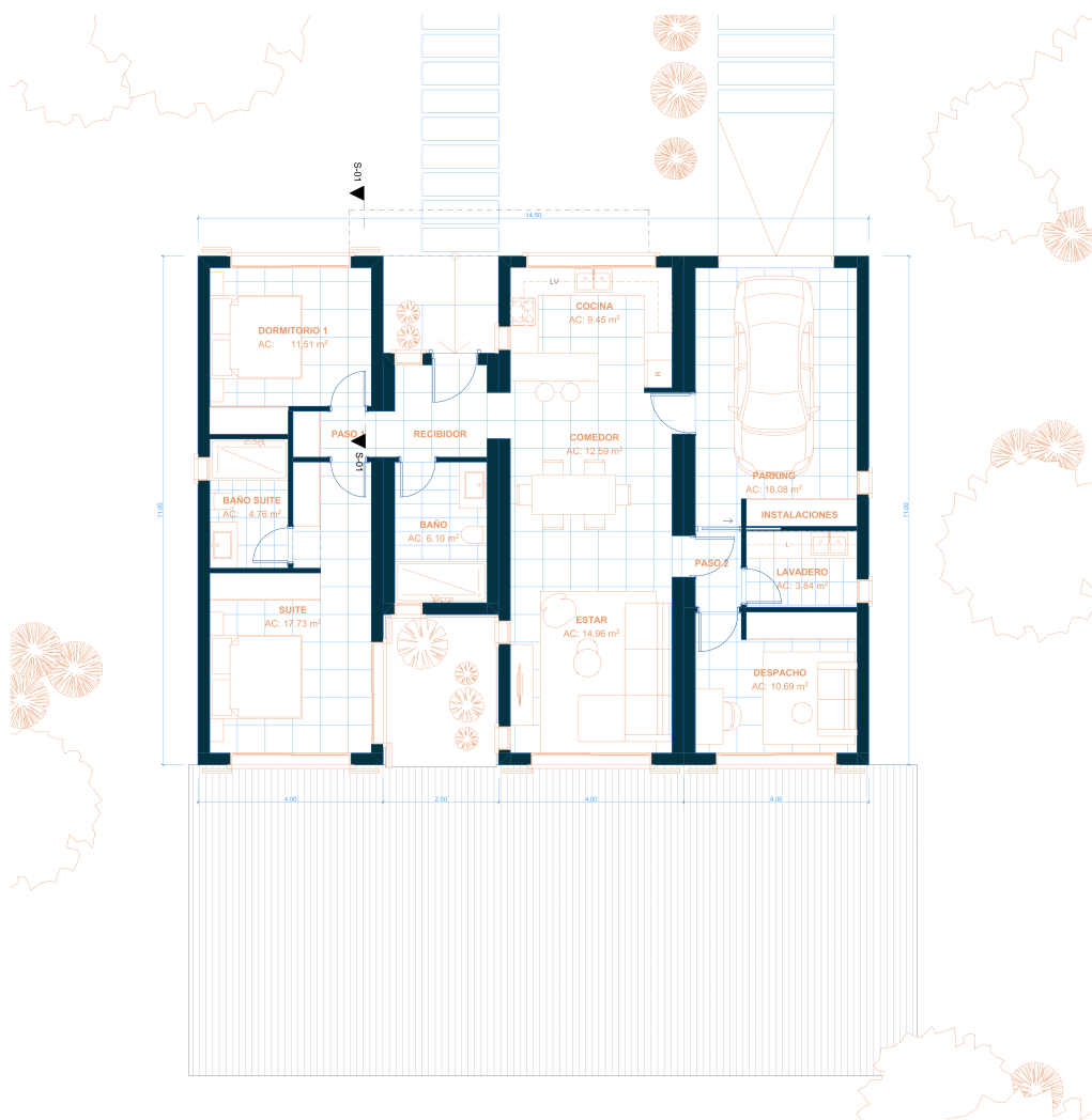
CASA REFUGIO EN EL MAR · PLANTA BAJA · ESC. 1:50
